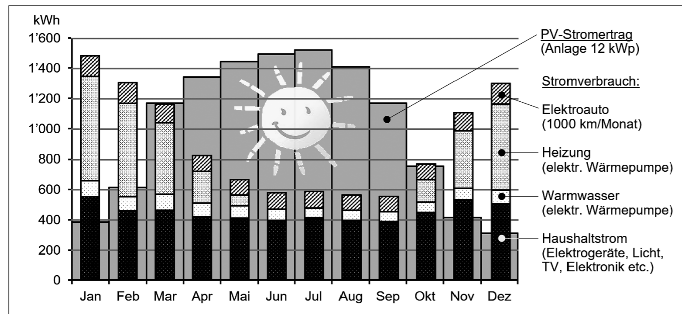
Abbildung 1: PV-Produktion und Stromverbrauch eines typischen EFH im Jahresverlauf, gemittelt aus Messdaten von 10 Jahren.
