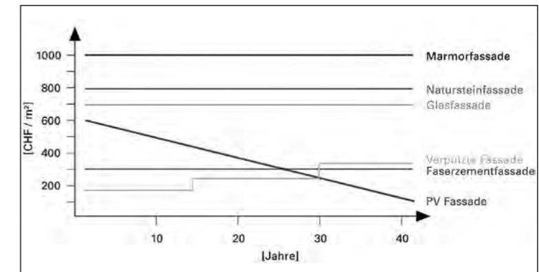
Grafik 3: Über einen Zeithorizont von 40 Jahren gesehen, ist eine PV-Fassade am kostengünstigsten (Grafik: Basler & Hofmann AG).
